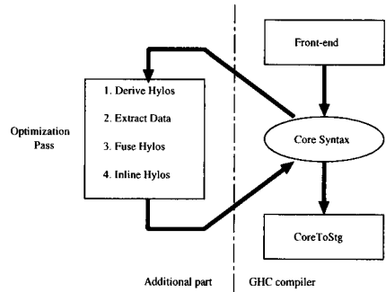
図 2 追加した変換部
