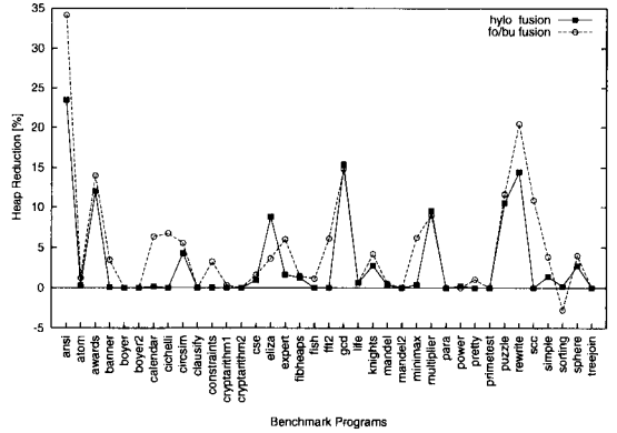
図 3 融合変換によるヒープ使用量の減少度
