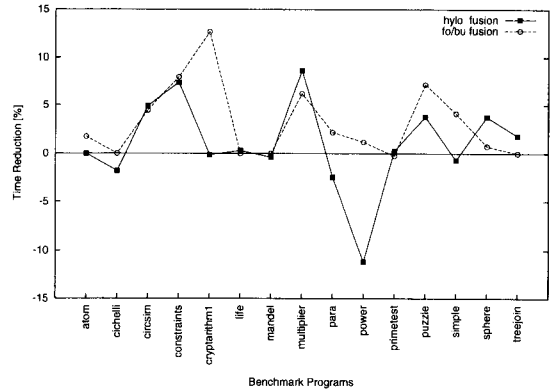
図 4 融合変換による実行時間の減少度
