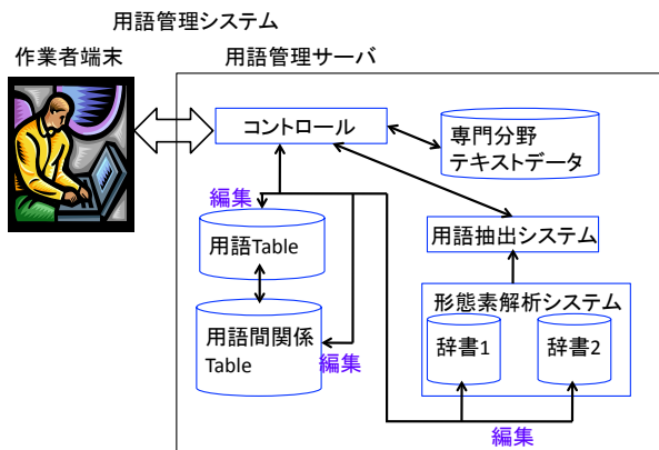
図 1: 用語管理システムの全体像
